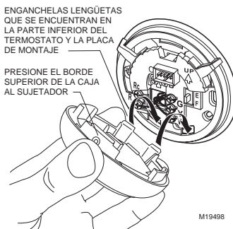
Figura 9. Montaje del termostato a la placa de fijación.
